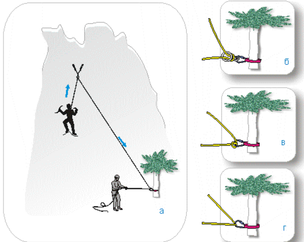
Мал.28. Загальна схема лазіння ТОП РОУП-страхування через пункт страхування .
