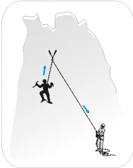
Мал.24. Загальна схема лазіння ТОП РОУП-страхування через бесідку .
