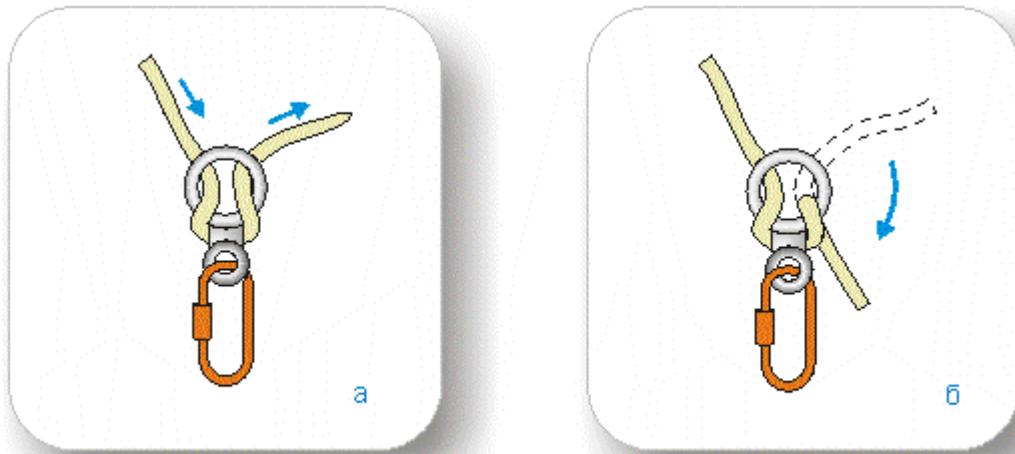
Мал.27. Вибирання та закріплення мотузки під час страхування.
