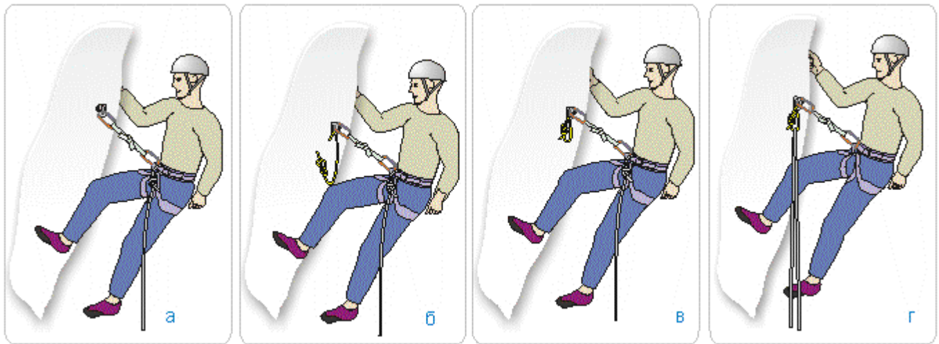
Мал.60.Організація спуску через петлю.
